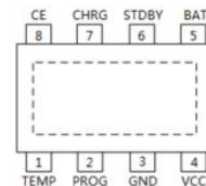
ESOP8
