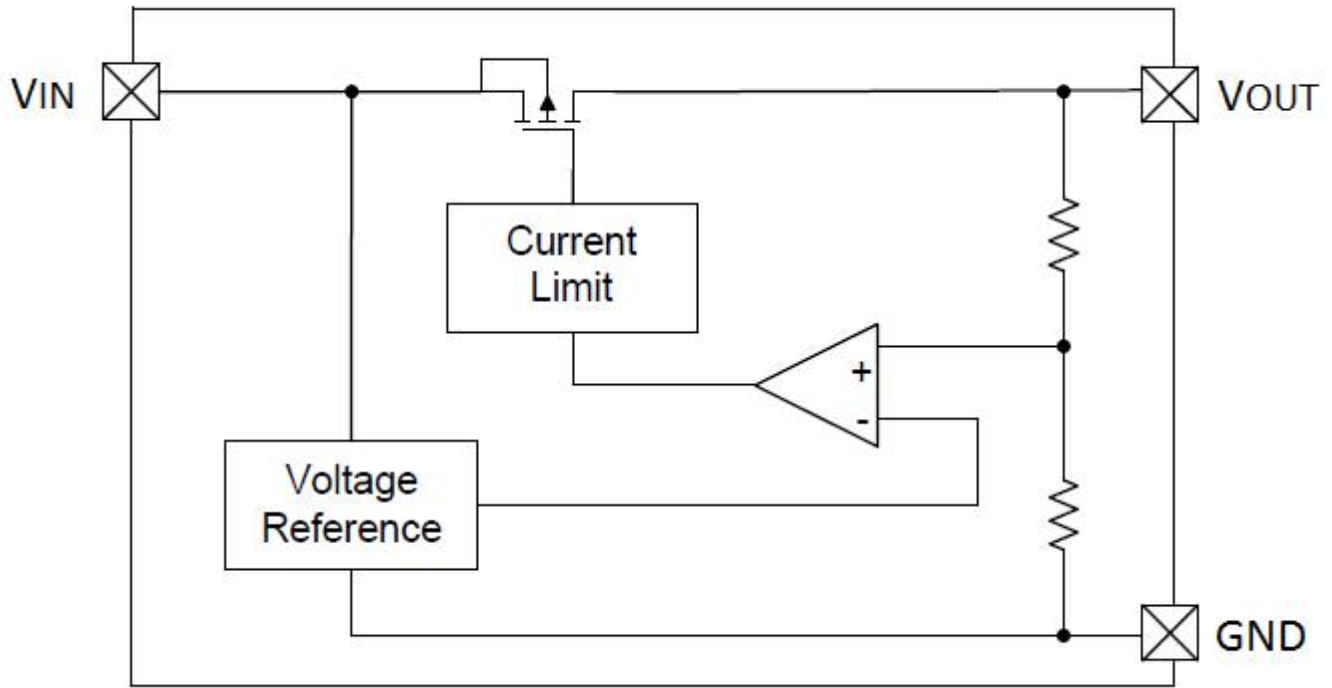
功能块框图
