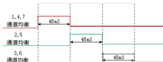
图二、电压判断和均衡动作时序图
