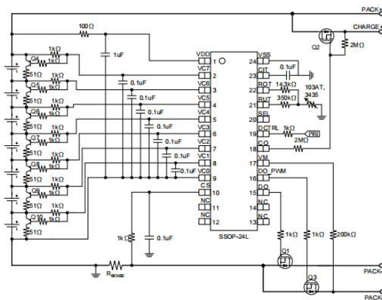
图三. 七串帶外部均衡应用线路
