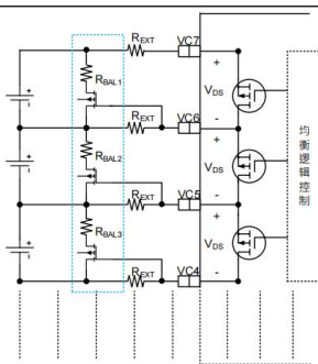
图一、外部均衡电路应用线路图
