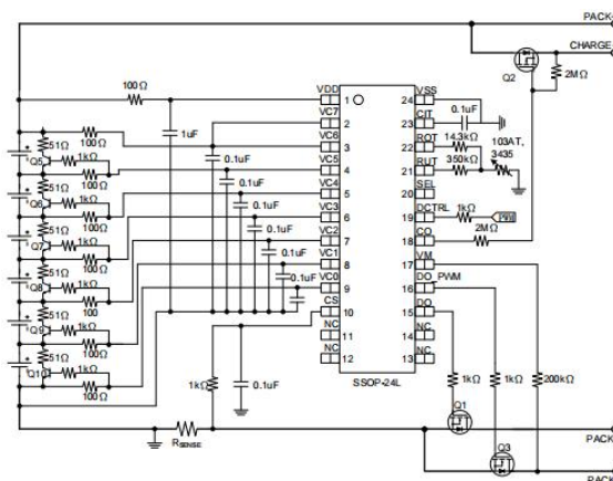
图四. 六串帶外部均衡应用线路
