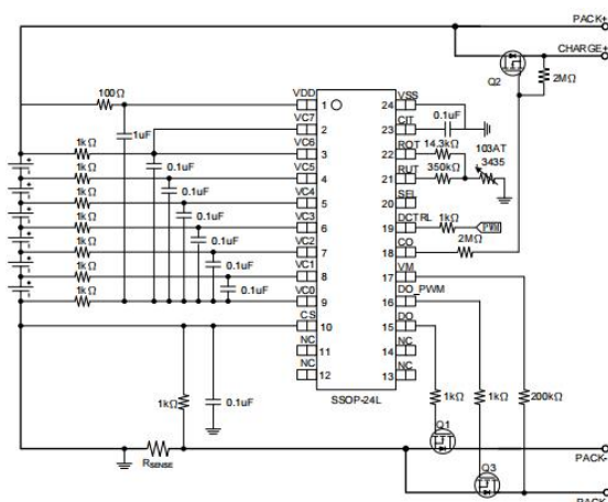
图五、七串不带外部均衡应用线路
