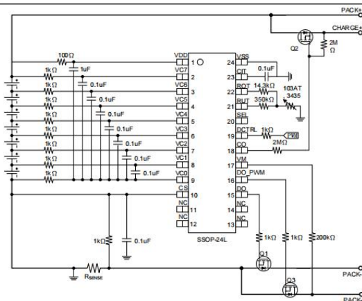
图五、七串不带外部均衡应用线路
