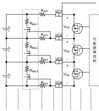
图一、外部均衡电路应用线路图
