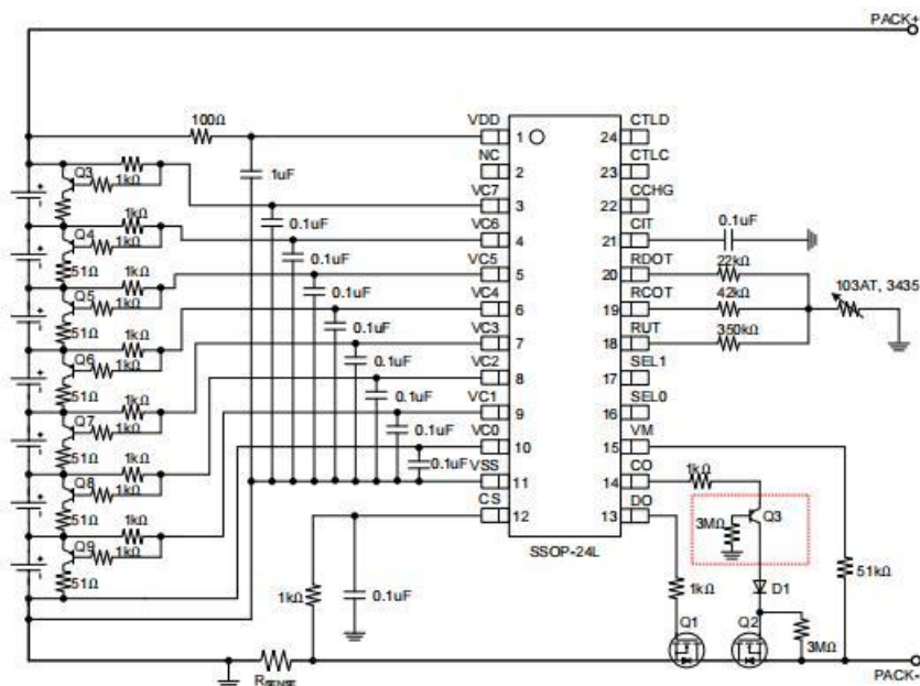
图三、七串带外部均衡应用线路
