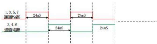
图二、电压判断和均衡动作时序图
