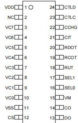
SSOP-24L
