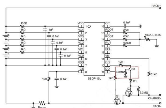
图五、四串不带外部均衡异口应用线路
