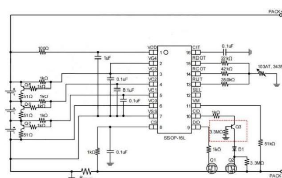
图六、三串带外部均衡应用线路
