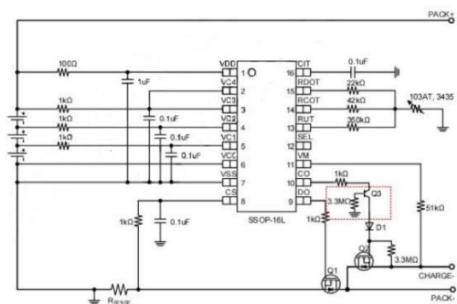
图八、三串不带外部均衡异口应用线路
