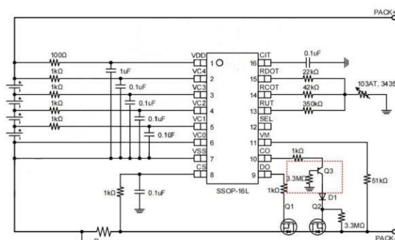
图四、四串不带外部均衡应用线路
