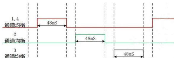
图二、电压判断和均衡动作时序图
