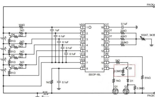
图三、四串带外部均衡应用线路
