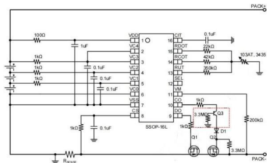
图七、三串不带外部均衡同口应用线路
