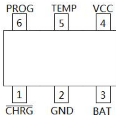
CL4267采用SOT-23-6L封装
