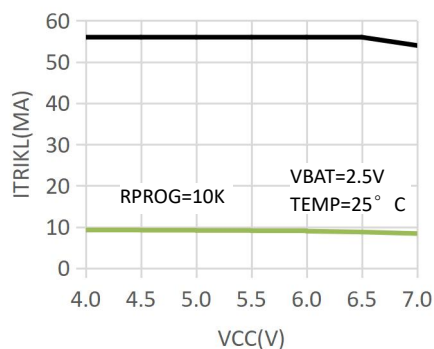
涓流充电电流与电源电压的关系曲线
