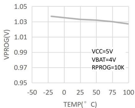
PROG引脚电压与温度的关系曲线
