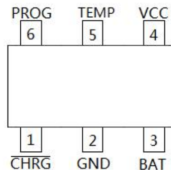
CL4267H采用SOT-23-6L封装
