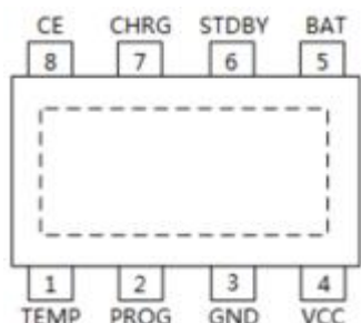
ESOP8
