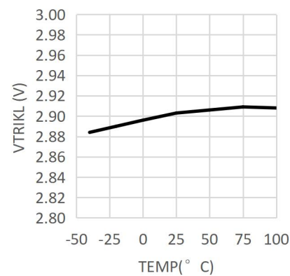
涓流充电门限电压与温度的关系曲线
