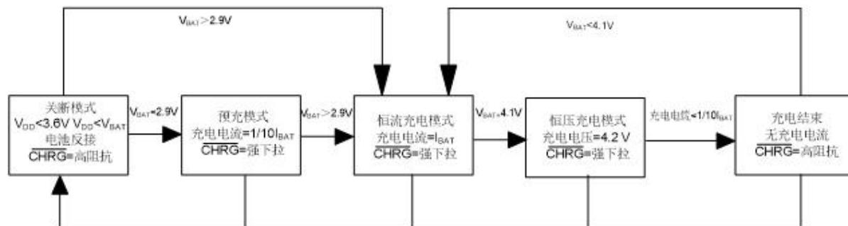
一个典型充电循环的状态图
