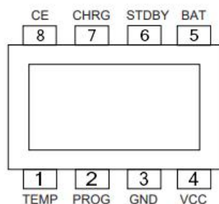
ESOP8L
