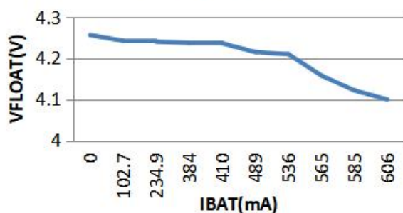
浮充电压与充电电流关系
