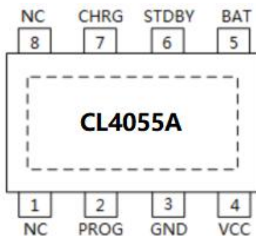
ESOP8
