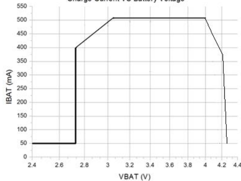
充电电压与充电电流关系
