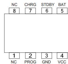
CL4055A采用ESOP8封装
