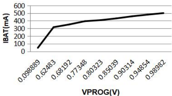
充电电流与PROG引脚电压的关系曲线
