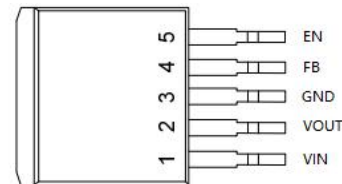
TO-263-5L
