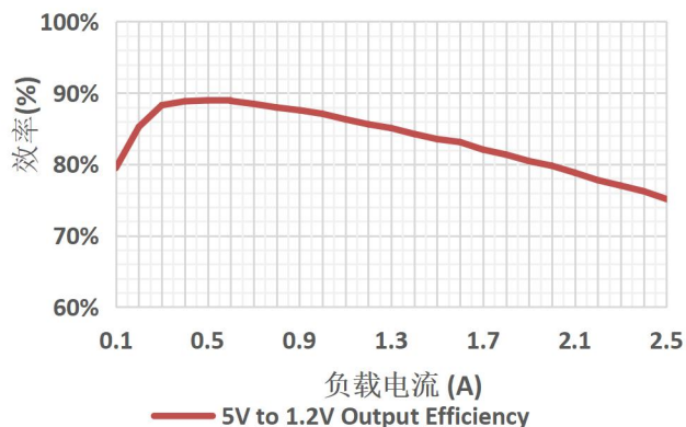
5V 转 1.2V 输出效率
