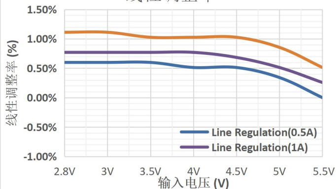
线性调整率
