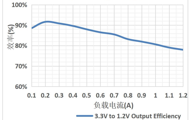
3.3V 转 1.2V 输出效率
