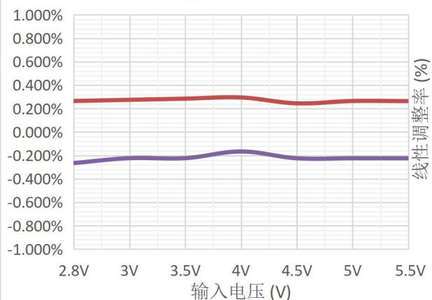
线性调整率
