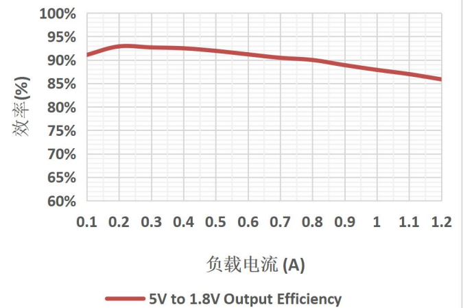
5V 转 1.8V 输出效率
