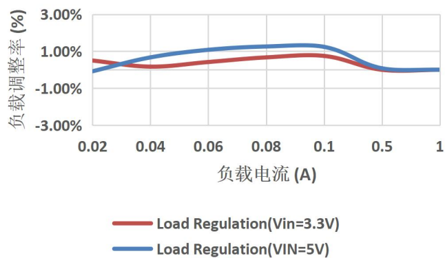
负载调整率
